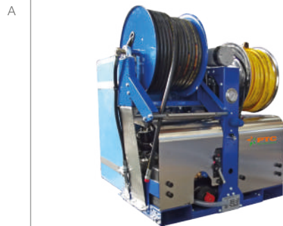
Version with electric powered hose reel Versione con avvolgitubo elettrico
